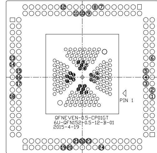
IC 脚位图
